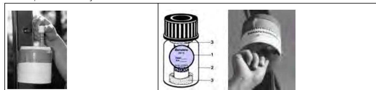
Exemple d'installation des tubes pour le dioxyde d'azote (gauche) et pour les tubes BTEX (droite).
